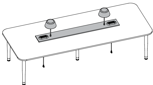
Chargeurs (ZNEP), chemin de table et lampes de table (ZNETL) Deux chargeurs aux extrémités et deux lampes vers l'intérieur
