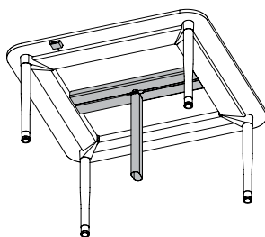
Cache-fils pour table d'atelier (ZNEW) et gestionnaire de câblage pour table d'atelier (ZNEC) Les câbles sont dissimulés.
