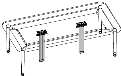
Gestionnaire de câblage pour table d'atelier (ZNEC) Les câbles sont dissimulés.
