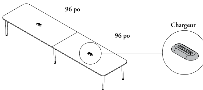
48 po x 192 po (P x La) Peut avoir 2 découpes pour chargeur
