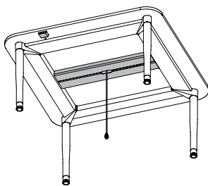
Cache-fils pour table d'atelier (ZNEW) Les câbles sont dissimulés sous la table, mais visibles au sol.
