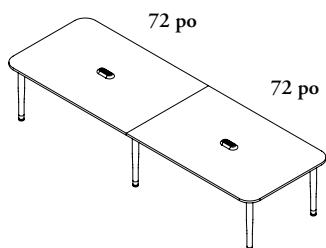
48 po x 144 po (P x La) Peut avoir 2 découpes pour chargeur
