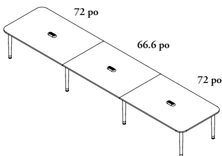
48 po x 216 po (P x La) Peut avoir 3 découpes pour chargeur
