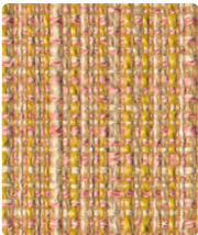
Quasar 4109-14
