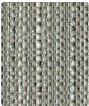
Allotrope 4109-04
